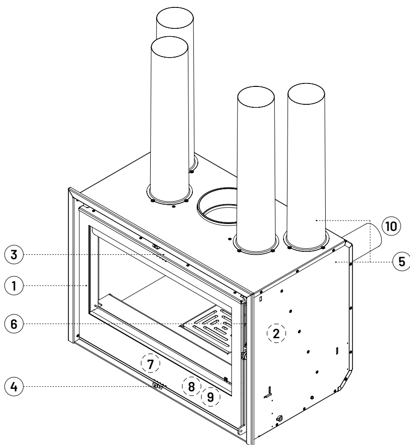
* Schéma explicatif : Modèle RCr80
